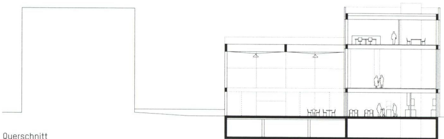
Querschnitt
