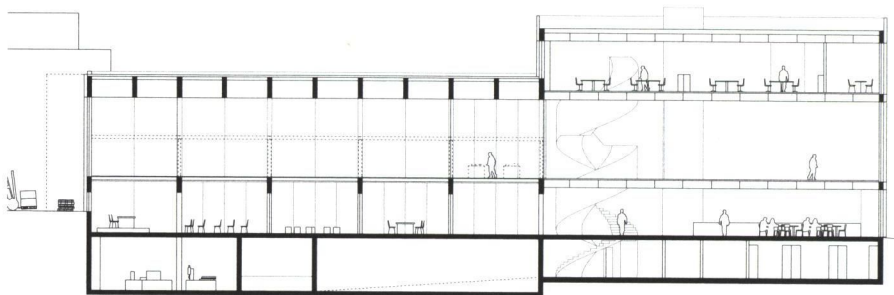
Längsschnitt
