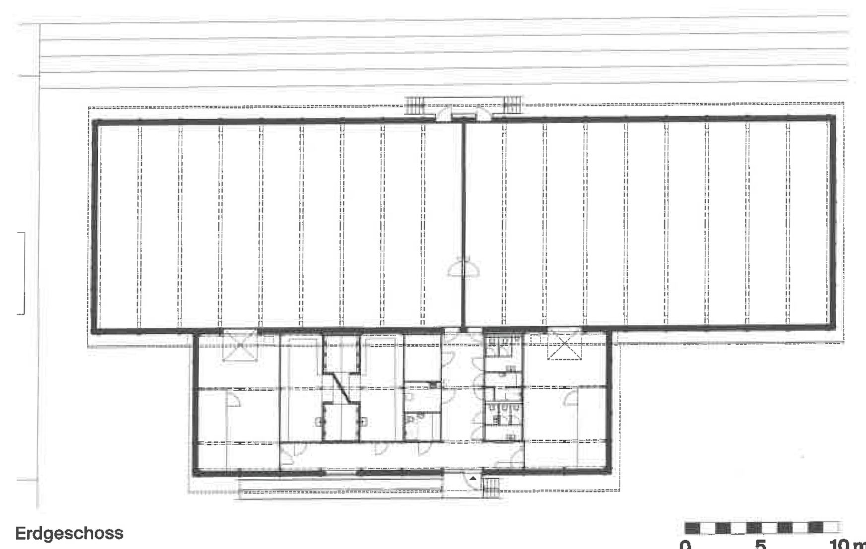
Erdgeschoss
