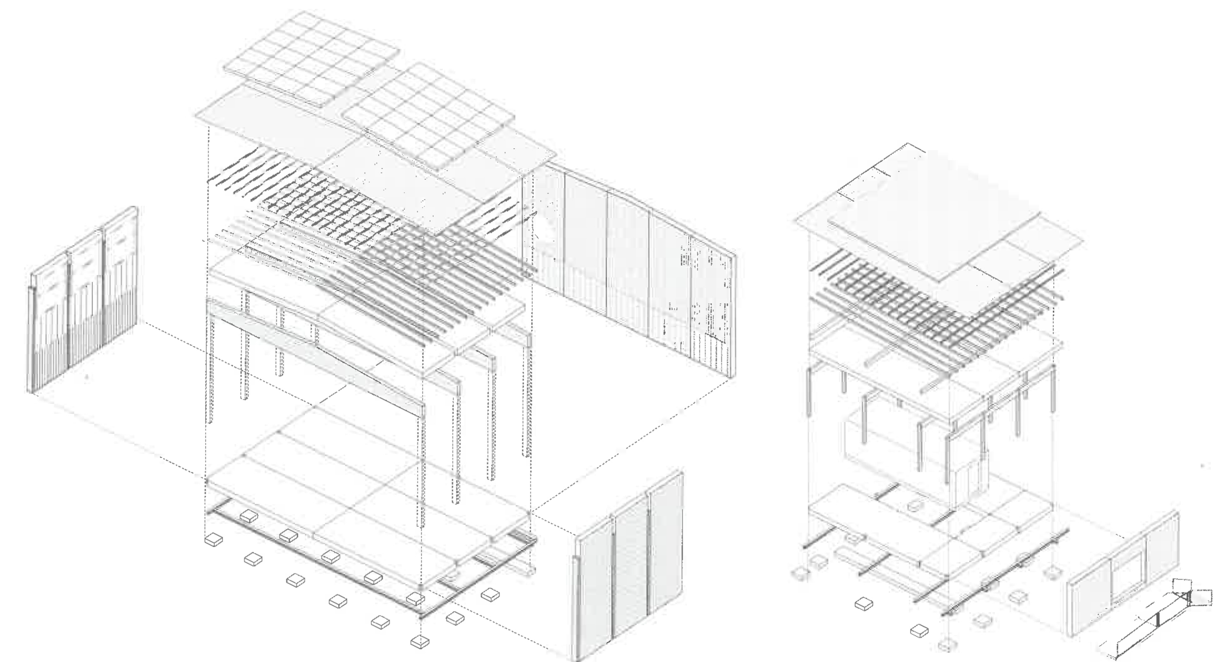
Konstruktions-Axonometrie der Sporthalle
