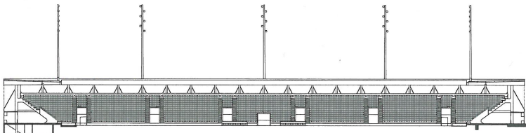
^17_Fussballstadion Arena, Längsschnitt.
