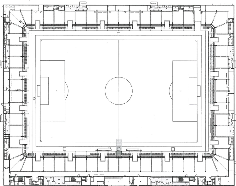
^17_Fussballstadion Arena, Grundriss Zugangsebene.
