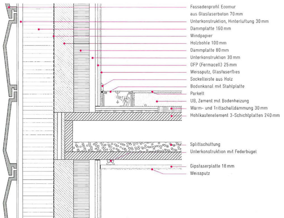
^ Detail Deckenanschluss-Fassade 1:10
