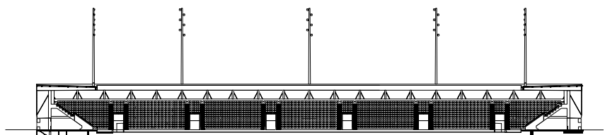
Längsschnitt
