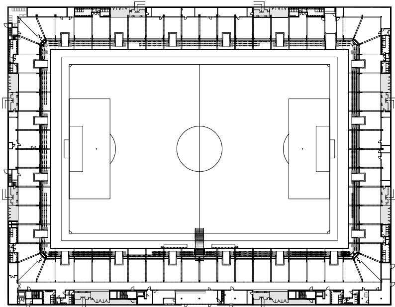
Erdgeschoss
