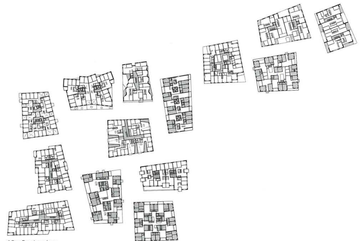
^ Das Regelgeschoss.
