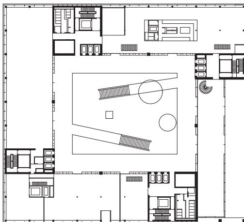
Erdgeschoss
