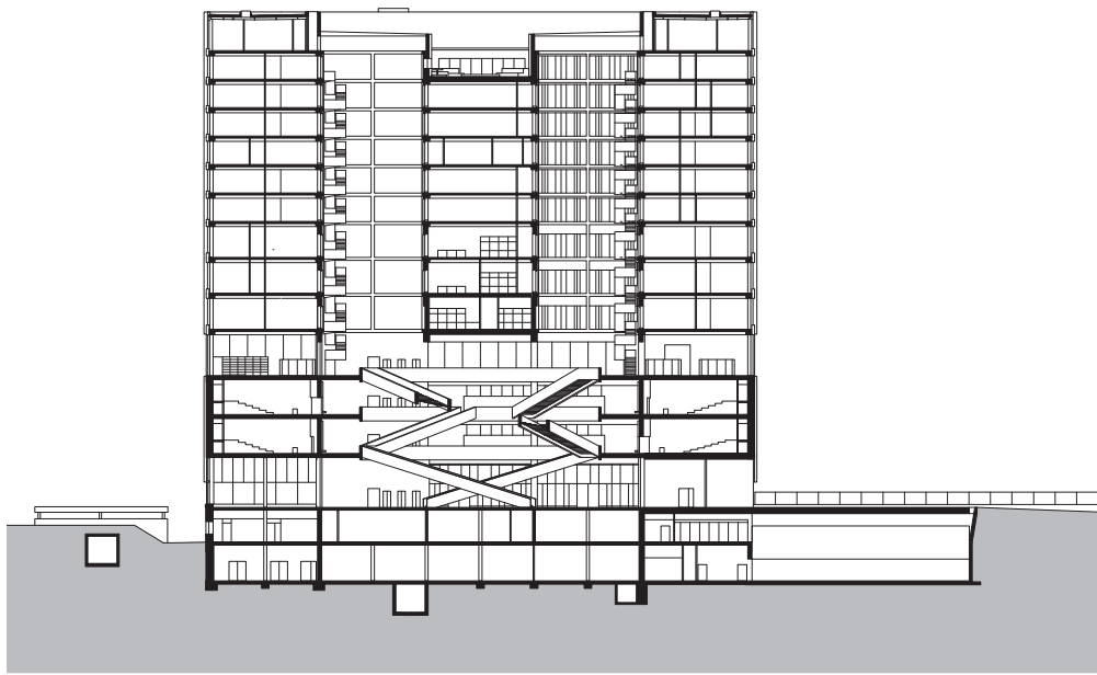
Querschnitt
