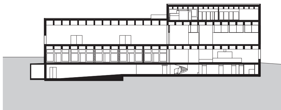
Längsschnitt
