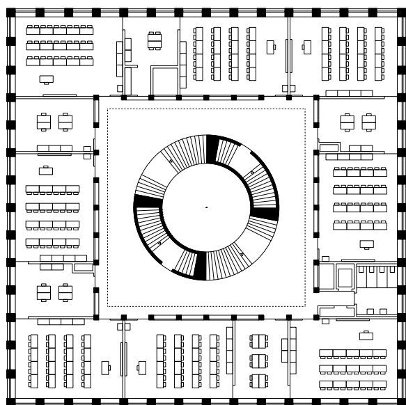
1. Obergeschoss
