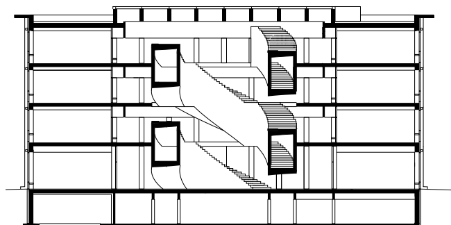
Schnitt
